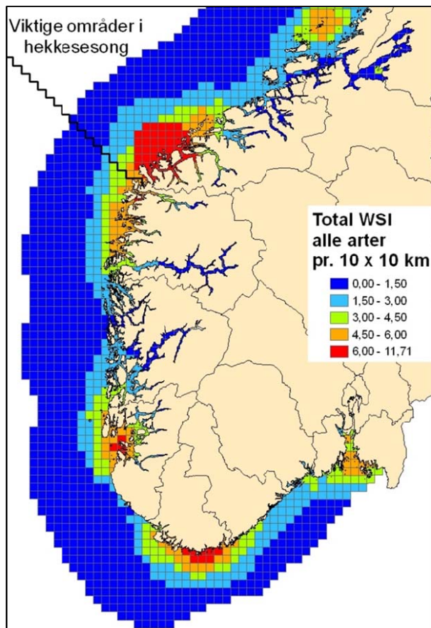
Figur 7.2 Samlekart for WSI summert for alle arter i Nordsjøen i sommersesongen, basert på kystdata. Avgrensningen for Nordsjøen er markert med svart linje. For hver 10x10 km. rute er den summerte verdien for alle inkluderte arter vist.
