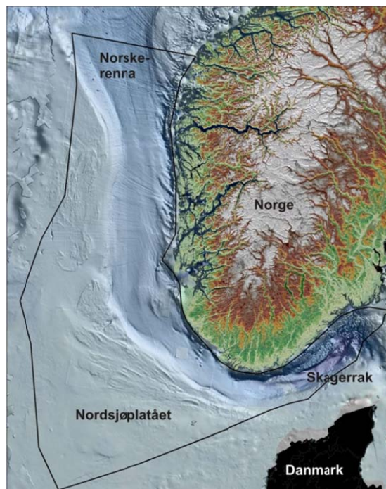
Figur 2.1 Utredningsområdets lokalisering og bunntopografi. Den tilstøtende kystsonen vil også bli utredet gjennom arbeidet. (Kilde: NGU/Statens kartverk)
